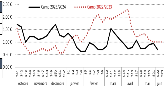
Evolution du prix moyen de tomate marocaine cal.67-82 marché St. Charles (€/kg)
